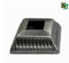
Основание баясины, арт. 8.6020 60x60x1мм, кв.20x20мм Вес: 0.04 кг Цена (за шт): 43 руб.
