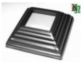
Основание балясины, арт. 13.321.02 90х90х1мм, кв.40х40мм Вес: 0.071 кг нет в наличии
