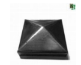
Заглушка на столб 50x50, арт. 15.054.02 50x50x1мм Вес: 0.036 кг Цена: 10,50 руб.
