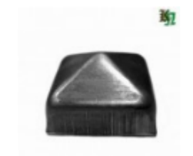
Заглушка на столб 40x40, арт. 15.053.02 40x40x1мм Вес: 0.02 кг Цена: 9 руб.
