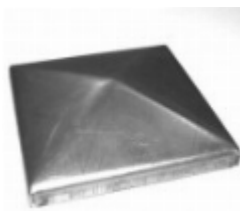
Заглушка, арт. 15.059 150x150x1мм Вес: 0.25 кг Цена: 96 руб.
