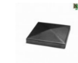
Заглушка на столб 60x60, арт. 15.055.36 60x60x1мм Вес: 0.03 кг Цена: 19 руб.
