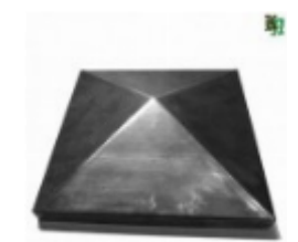
Заглушка на столб 80x80, арт. 15.056.02 80x80x1мм Вес: 0.079 кг Цена: 21 руб.
