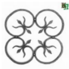
Розетка, арт. 174 470x470мм, кв.10x10мм Вес: 2.4 кг Цена: 640 руб.
