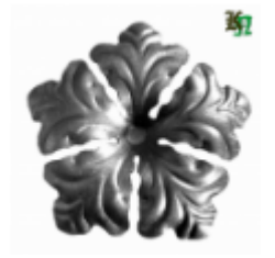
Цветок, арт. 5179.03 д=130x2мм Вес: 0.16 кг Цена (за шт): 70 руб.
