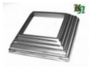
Основание блясины, арт. 13.380.01 122x122x1мм, кв.80x80мм Вес: 0.11 кг Цена: 50 руб.
